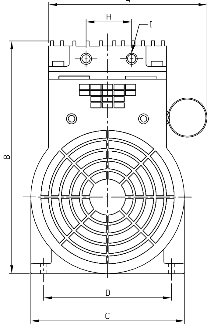
DP-200V Dimension (mm)
